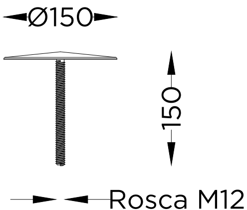
ALÇADO LATERAL SIDE VIEW
