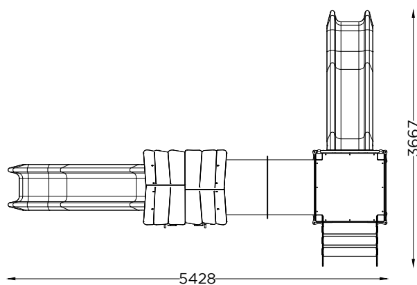
PLANTA PLAN
