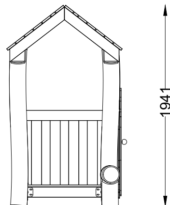
ALÇADO LATERAL SIDE VIEW
