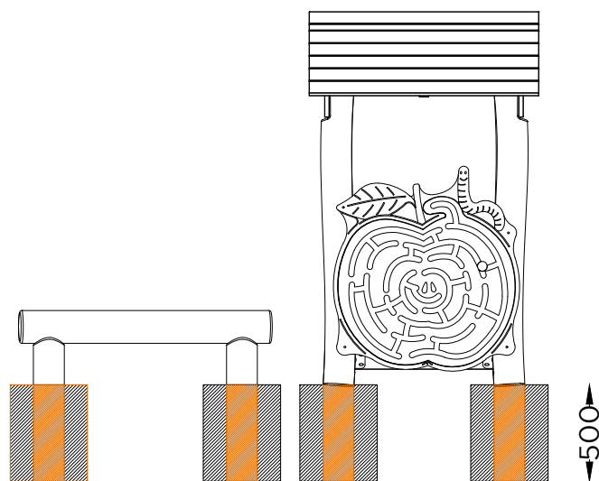
ALÇADO FRONTAL . ESQUEMA DE FIXAÇÃO FRONT VIEW . INSTALLATION PLAN
