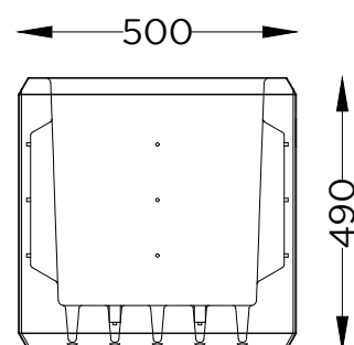
ALÇADO FRONTAL FRONT VIEW
