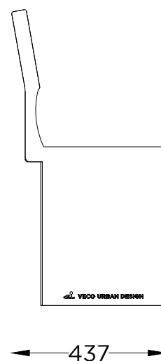
ALÇADO LATERAL SIDE VIEW
