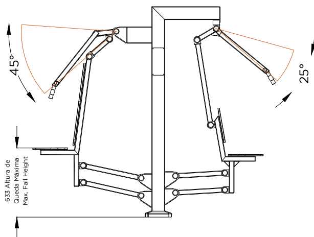
ALÇADO FRONTAL FRONT VIEW
