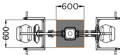
PLANTA . ESQUEMA DE FIXAÇÃO PLAN . INSTALLATION PLAN
