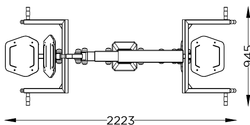
PLANTA PLAN
