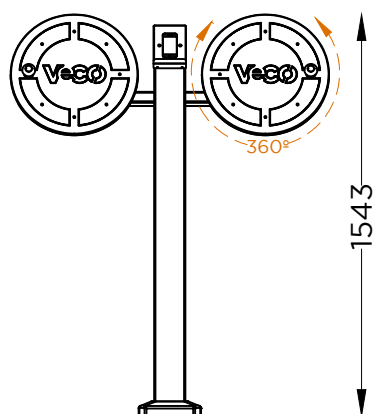
ALÇADO FRONTAL FRONT VIEW
