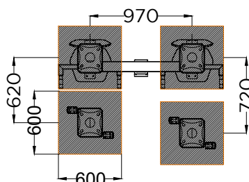
PLANTA . ESQUEMA DE FIXAÇÃO PLAN . INSTALLATION PLAN
