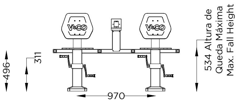
ALÇADO LATERAL SIDE VIEW
