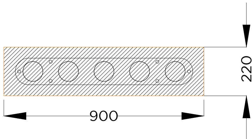
PLANTA . ESQUEMA DE FIXAÇÃO PLAN . INSTALLATION PLAN
