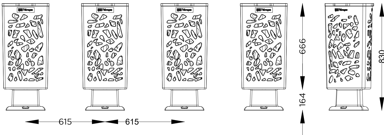
ALÇADO LATERAL SIDE VIEW
