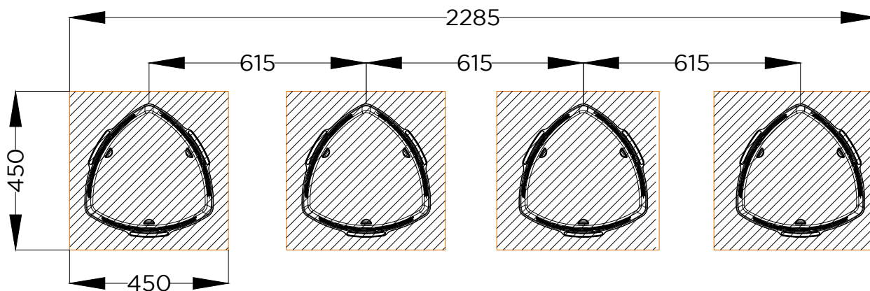
PLANTA . ESQUEMA DE FIXAÇÃO PLAN . INSTALLATION PLAN
