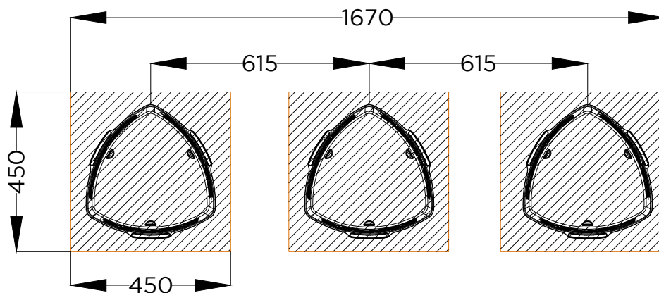
PLANTA . ESQUEMA DE FIXAÇÃO PLAN . INSTALLATION PLAN
