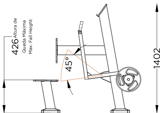
ALÇADO LATERAL SIDE VIEW
