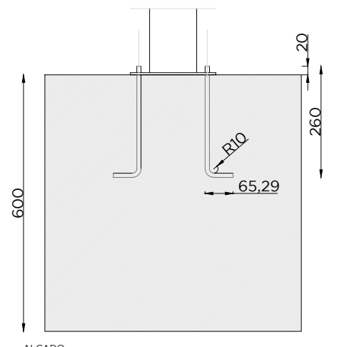
ALÇADO
