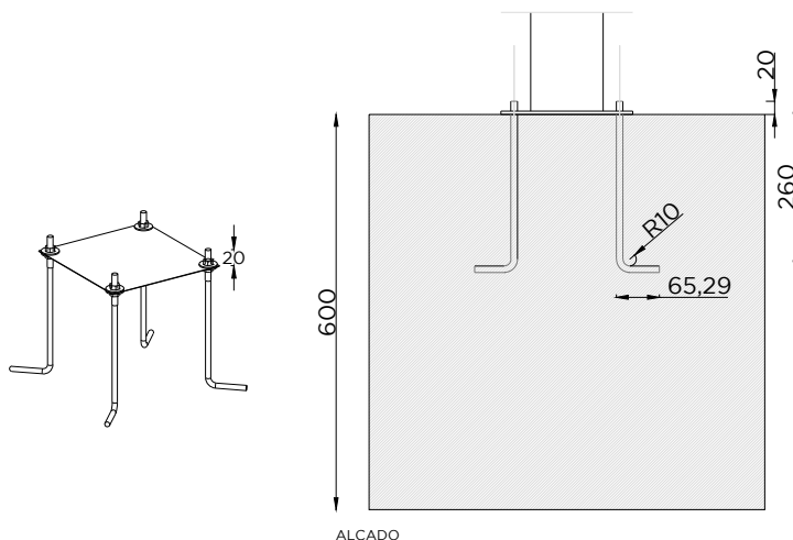
ALÇADO
