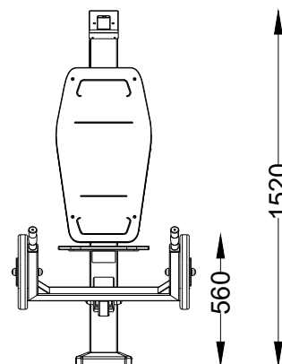
ALÇADO FRONTAL FRONT VIEW
