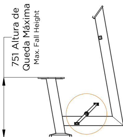
ALÇADO LATERAL SIDE VIEW
