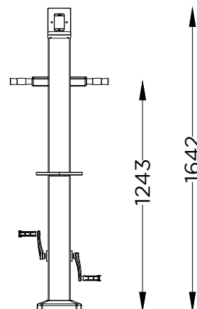
ALÇADO FRONTAL FRONT VIEW
