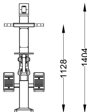
ALÇADO FRONTAL FRONT VIEW
