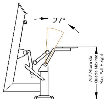
ALÇADO LATERAL SIDE VIEW
