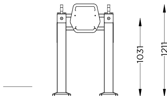
ALÇADO FRONTAL FRONT VIEW
