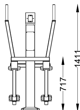
ALÇADO FRONTAL FRONT VIEW
