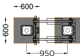
PLANTA . ESQUEMA DE FIXAÇÃO PLAN . INSTALLATION PLAN
