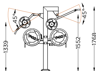
ALÇADO LATERAL SIDE VIEW
