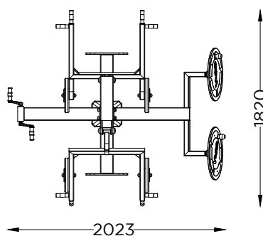
PLANTA PLAN
