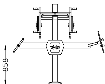
ALÇADO FRONTAL FRONT VIEW
