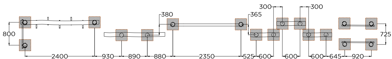
PLANTA . ESQUEMA DE FIXAÇÃO PLAN . INSTALLATION PLAN
