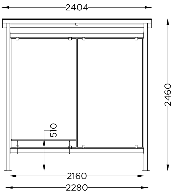
ALÇADO LATERAL SIDE VIEW
