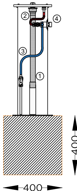
PLANTA . ESQUEMA DE FIXAÇÃO PLAN . INSTALLATION PLAN
