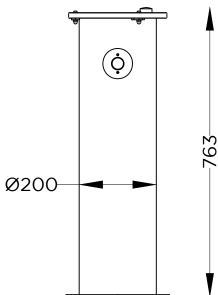
ALÇADO LATERAL SIDE VIEW
