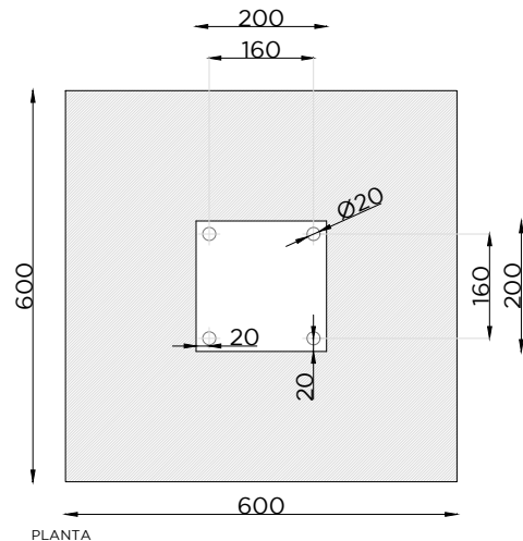
PLANTA
