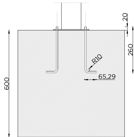
ALÇADO
