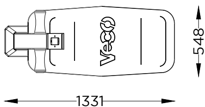
PLANTA PLAN
