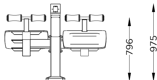
ALÇADO FRONTAL FRONT VIEW
