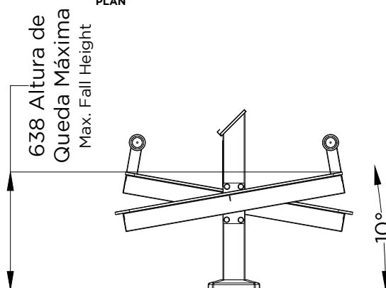
ALÇADO LATERAL SIDE VIEW
