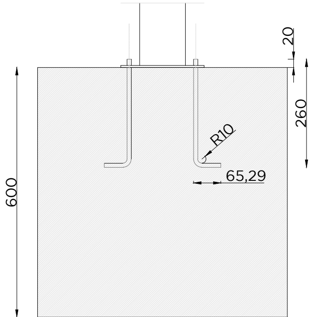
ALÇADO
