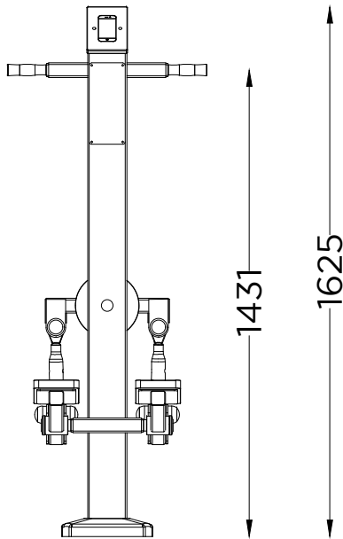
ALÇADO FRONTAL FRONT VIEW
