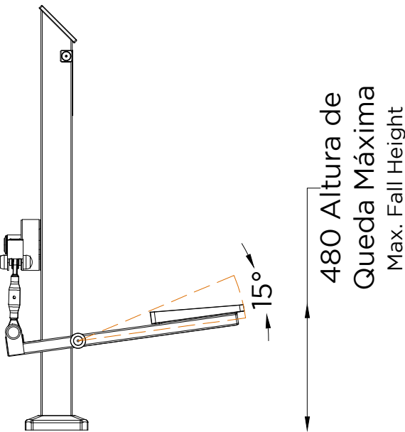
ALÇADO LATERAL SIDE VIEW
