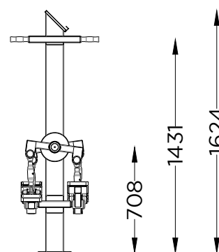
ALÇADO LATERAL SIDE VIEW
