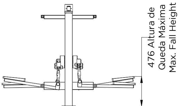
ALÇADO FRONTAL FRONT VIEW
