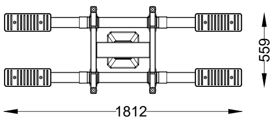
PLANTA PLAN
