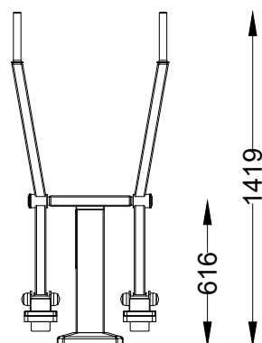
ALÇADO FRONTAL FRONT VIEW
