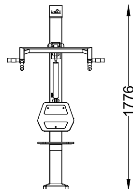
ALÇADO FRONTAL FRONT VIEW
