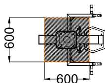
PLANTA . ESQUEMA DE FIXAÇÃO PLAN . INSTALLATION PLAN
