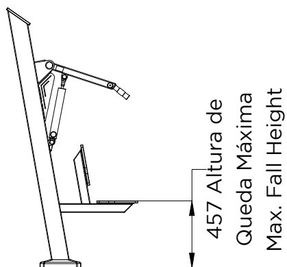
ALÇADO LATERAL SIDE VIEW
