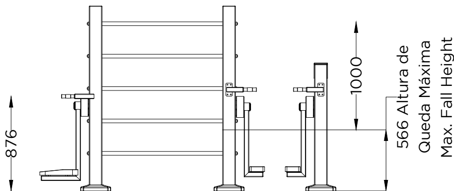
ALÇADO FRONTAL FRONT VIEW
