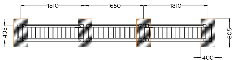
PLANTA . ESQUEMA DE FIXAÇÃO PLAN . INSTALLATION PLAN
