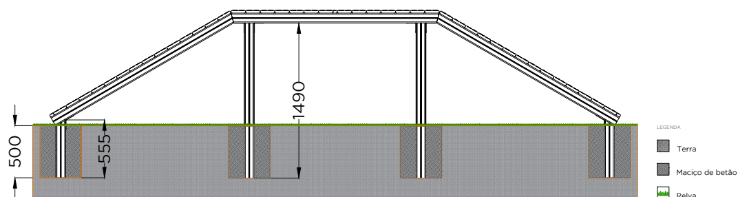
ALÇADO FRONTAL . ESQUEMA DE FIXAÇÃO FRONT VIEW . INSTALLATION PLAN
