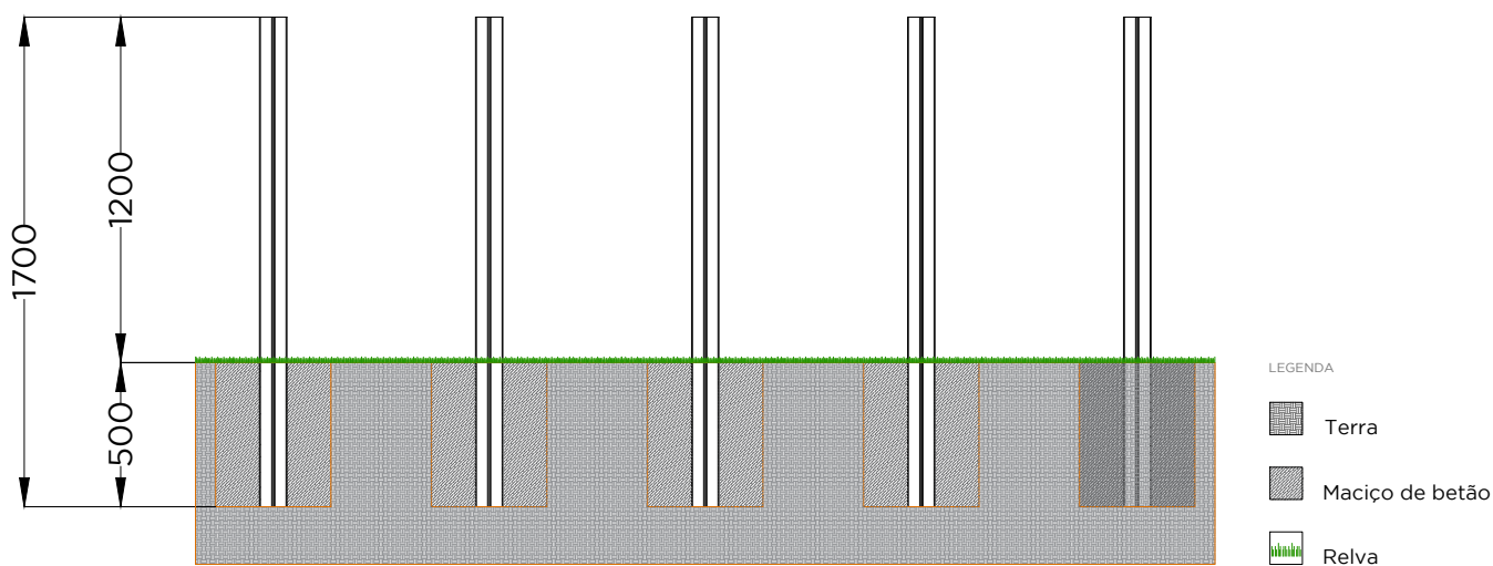
ALÇADO FRONTAL . ESQUEMA DE FIXAÇÃO FRONT . INSTALLATION PLAN
