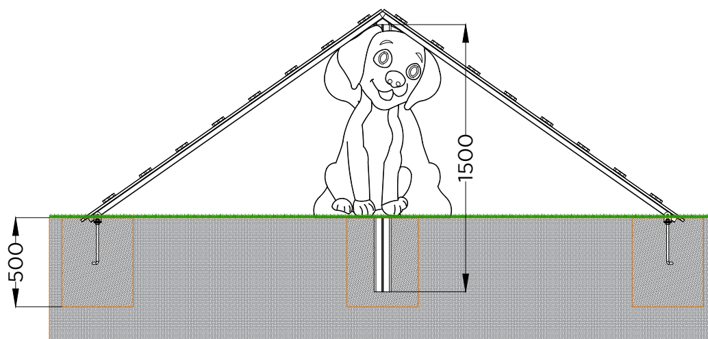
ALÇADO FRONTAL . ESQUEMA DE FIXAÇÃO FRONT VIEW . INSTALLATION PLAN
