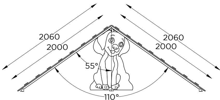
ALÇADO FRONTAL FRONT VIEW
