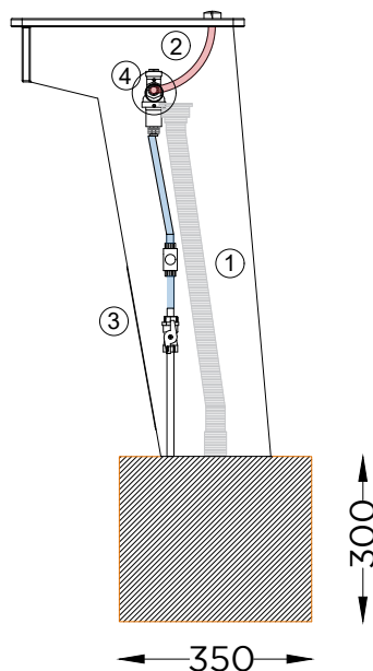
ALÇADO LATERAL SIDE VIEW
