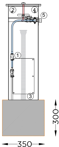
ALÇADO FRONTAL FRONT VIEW
