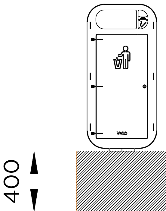
ALÇADO FRONTAL . ESQUEMA DE FIXAÇÃO FRONT VIEW . INSTALLATION PLAN
