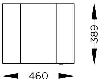
PLANTA PLAN
