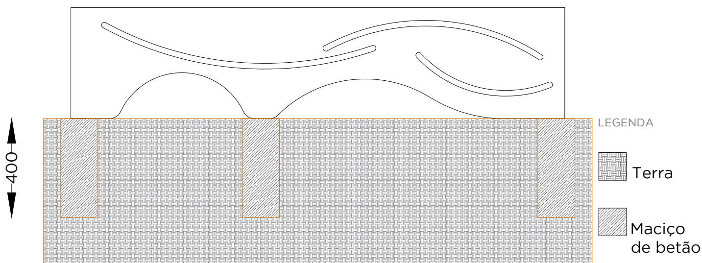
ALÇADO FRONTAL . ESQUEMA DE FIXAÇÃO FRONT VIEW . INSTALLATION PLAN
