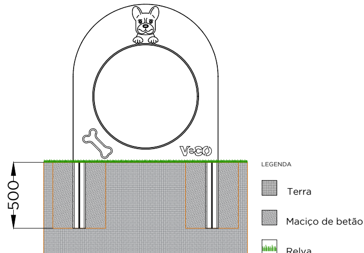
ALÇADO FRONTAL . ESQUEMA DE FIXAÇÃO FRONT VIEW . INSTALLATION PLAN
