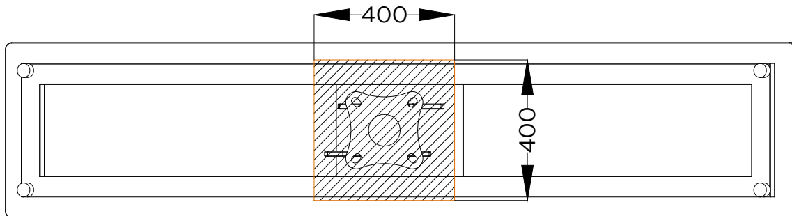
PLANTA . ESQUEMA DE FIXAÇÃO PLAN . INSTALLATION PLAN
