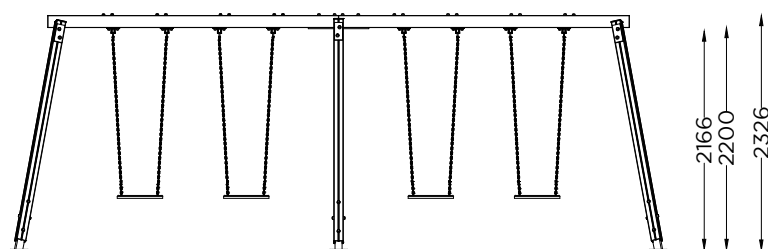
ALÇADO FRONTAL FRONT VIEW
