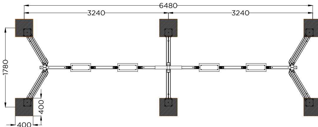
PLANTA . ESQUEMA DE FIXAÇÃO EM AREIA PLAN . SAND FIXATION SCHEME.
