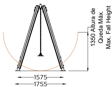
ALÇADO LATERAL SIDE VIEW
