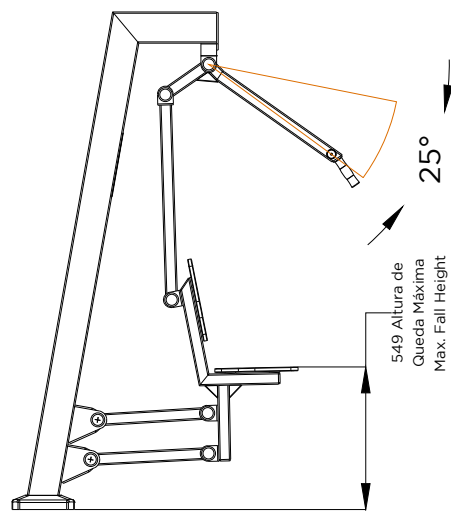
ALÇADO LATERAL SIDE VIEW
