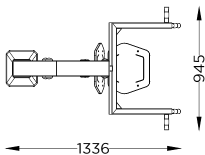
PLANTA PLAN
