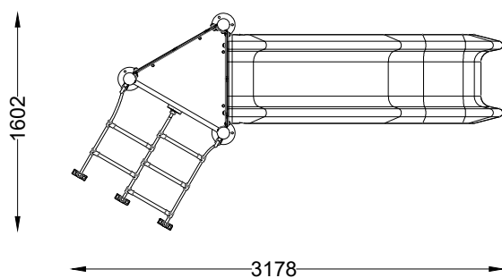
PLANTA PLAN
