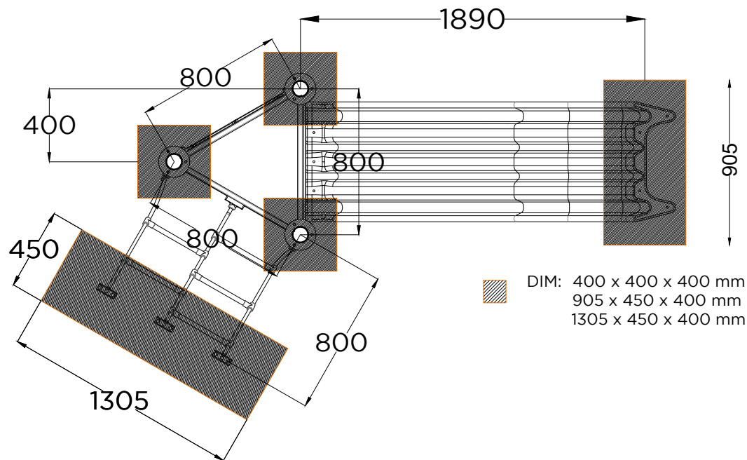
PLANTA . ESQUEMA DE FIXAÇÃO PLAN . INSTALLATION PLAN
