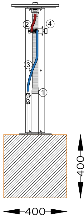
PLANTA . ESQUEMA DE FIXAÇÃO PLAN . INSTALLATION PLAN
