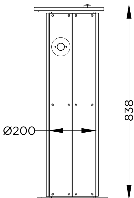
ALÇADO LATERAL SIDE VIEW
