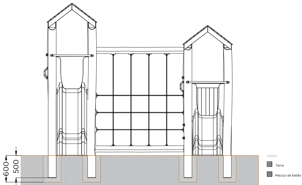
ALÇADO LATERAL . ESQUEMA DE FIXAÇÃO SIDE VIEW . INSTALLATION PLAN
