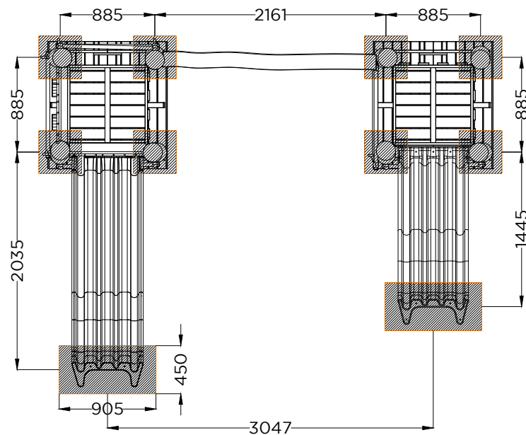
PLANTA . ESQUEMA DE FIXAÇÃO PLAN . INSTALLATION PLAN
