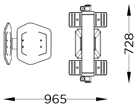
PLANTA PLAN
