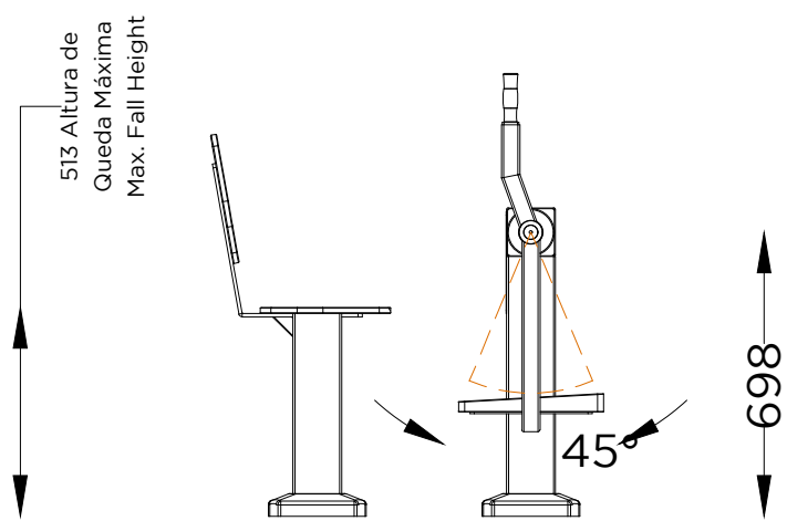
ALÇADO LATERAL SIDE VIEW
