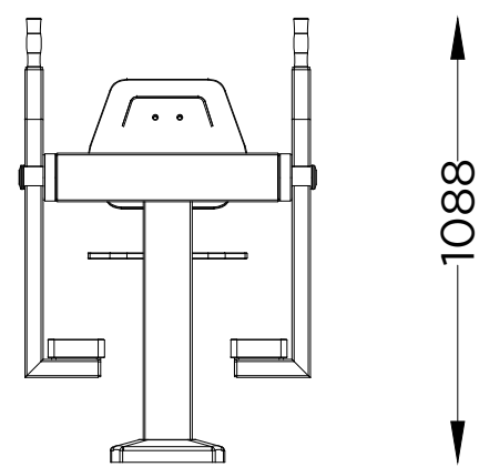
ALÇADO FRONTAL FRONT VIEW
