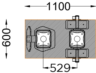
PLANTA . ESQUEMA DE FIXAÇÃO PLAN . INSTALLATION PLAN
