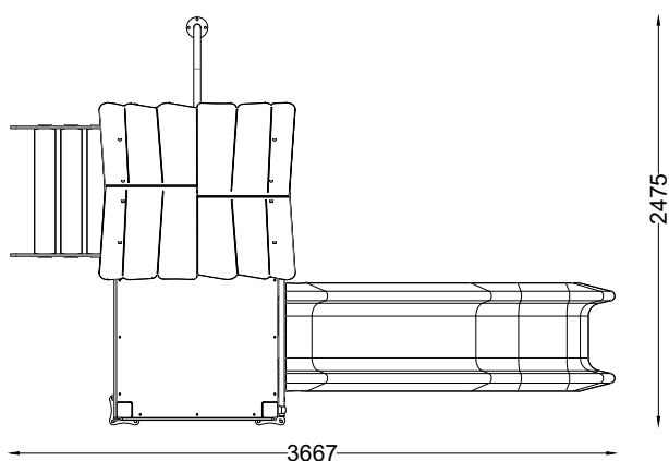
PLANTA PLAN
