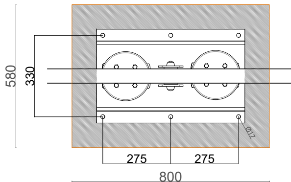
PLANTA . ESQUEMA DE FIXAÇÃO PLAN . INSTALLATION PLAN
