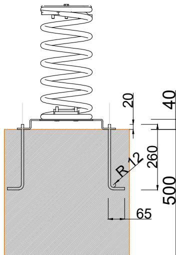
ALÇADO . ESQUEMA DE FIXAÇÃO SIDE VIEW . INSTALLATION PLAN
