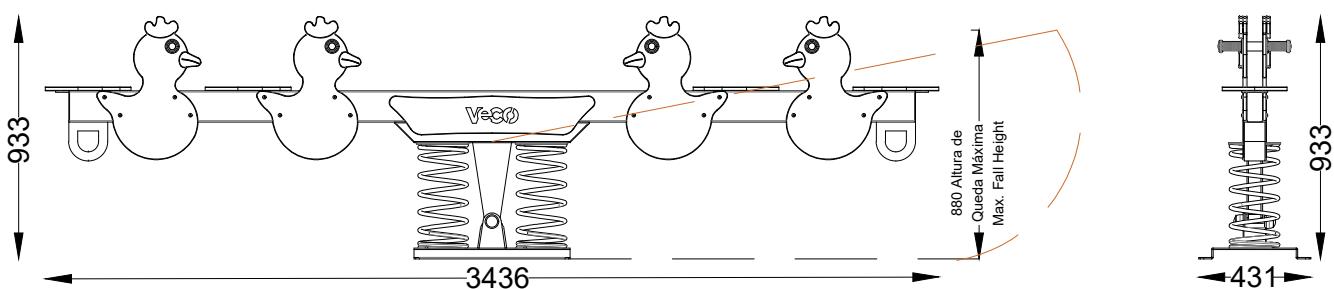
ALÇADO LATERAL SIDE VIEW
