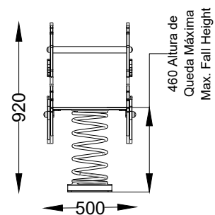
ALÇADO FRONTAL FRONT VIEW
