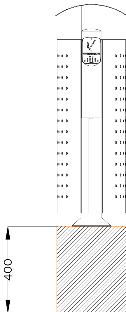
ALÇADO LATERAL . ESQUEMA DE FIXAÇÃO SIDE VIEW . INSTALLATION PLAN
