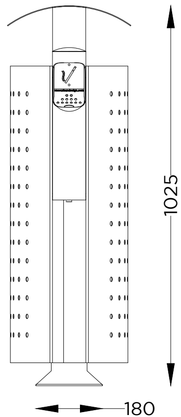
ALÇADO LATERAL SIDE VIEW
