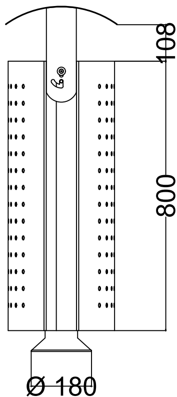
ALÇADO LATERAL SIDE VIEW
