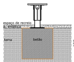
ESQUEMA DE FIXAÇÃO POR SAPATA
