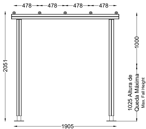
ALÇADO FRONTAL FRONT VIEW
